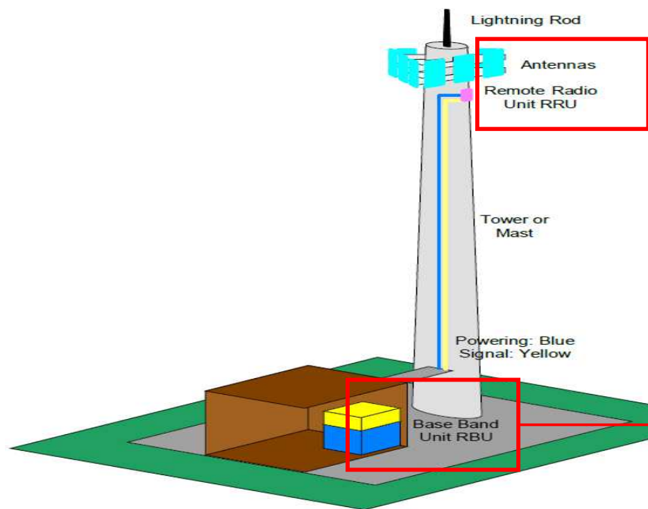
4G基站简图
