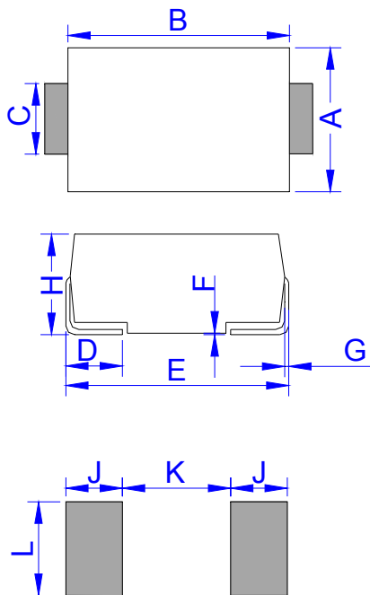
DO-214AC (SMA)
